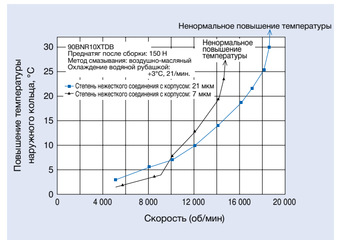
Рис. 5.3 Влияние зазора между подшипником и корпусом на предельную скорость
