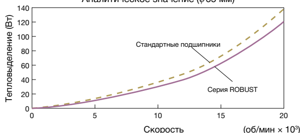
Тепловыделение при смазывании консистентной смазкой Аналитическое значение ( \phi 65 мм)
