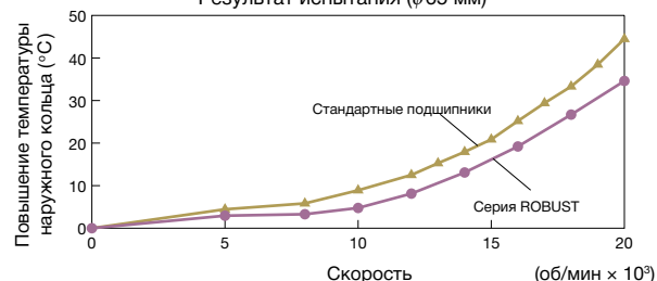
Повышение температуры наружного кольца при смазывании консистентной смазкой Результат испытания ( \phi 65 мм)
