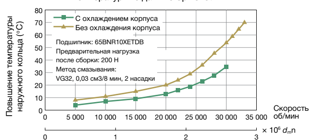
Температурные данные Spinshot™ II
