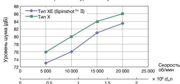
Сравнение уровней шума
