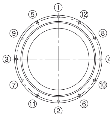
Рис. 1 Порядок затяжки
