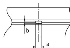
Детальный вид отверстия для смазки
