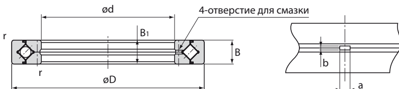
Детальный вид отверстия для смазки
