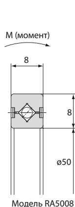
Подшипник с перекрестными роликами
