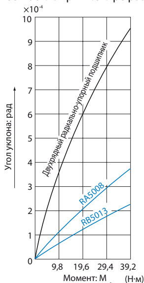
Диаграмма жёсткости моментов
