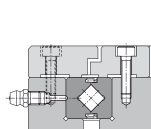
с. Внутренние и наружные кольца закрепляются в том же направлении в шарнирном блоке (с установленными уплотнениями)
