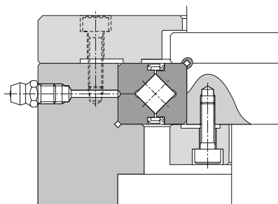
б. Вращение внутреннего кольца в шарнирном блоке (с установленными уплотнениями)
