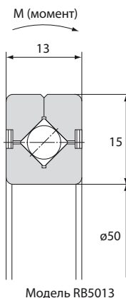
Подшипник с перекрестными роликами
