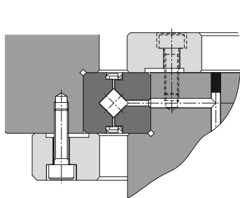
а. Вращение наружного кольца в шарнирном блоке:
