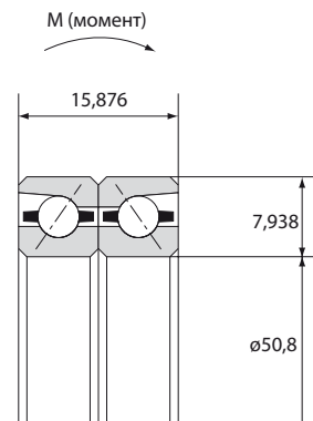
Радиально-упорный шарикоподшипник
