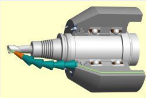
Опция TSCW2 - дополнительный подвод охлаждающего средства
