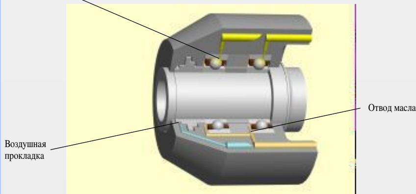
AI: Впрыскивание воздушно-масляного тумана для наилучшей эксплуатации
