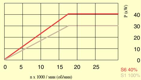
HF 170.5 AI22 - асинхронный мотор
