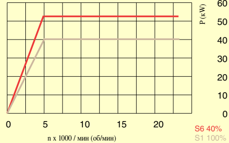
HF 230.4 AI20 Δ-соединение 380 V / 119 A
