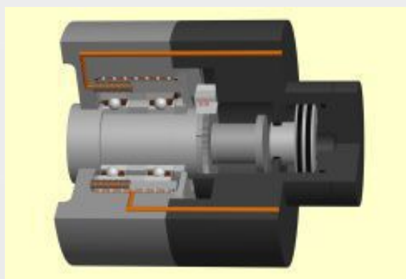
Управляемый в зависимости от скорости вращения гидравлический преднатяг. Преимущество: дополнительное демпфирование для увеличения срока службы подшипников и инструмента.
