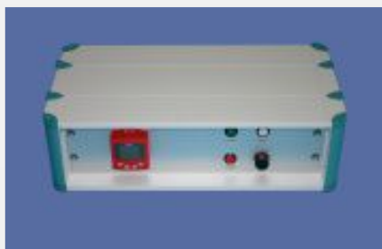
Регулятор оборотов для малых шпинделей HF 25, HF 33, HF 45 или HFK 90.1, HFK95
