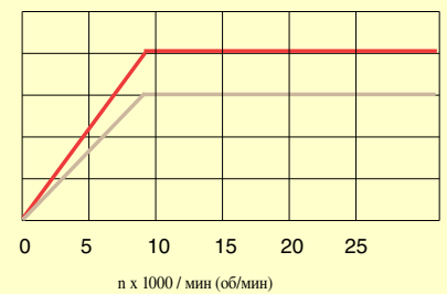
HF 170.5 AI22 - синхронный мотор
