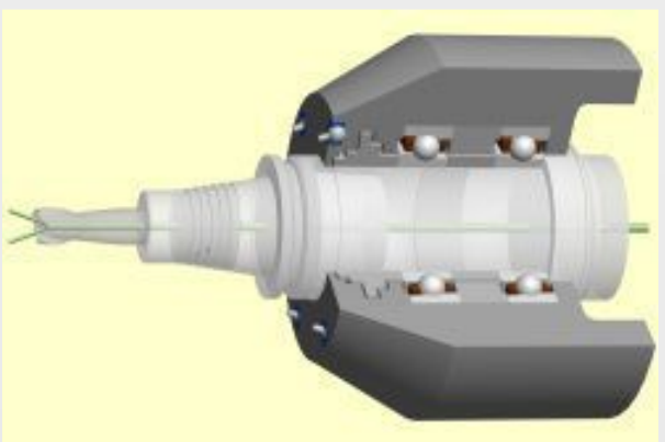
Опция W - подвод СОЖ через центр
