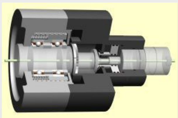
Задняя сторона шпинделя с муфтой для подачи СОЖ
