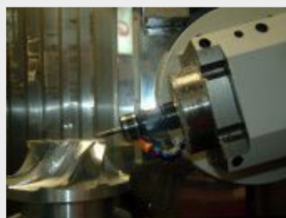
Пятиосевое фрезерование турбинных лопаток на HF120
