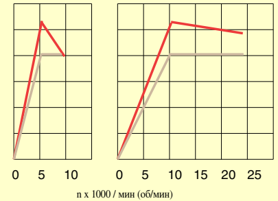
HF 230.4 AI20 Y-Δ-соединение 380 V / 74 A
